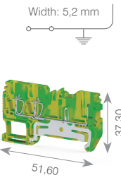
CTP 2.5ET
