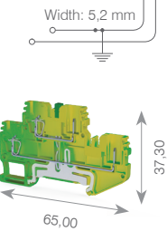
CTP 2.5-2T
