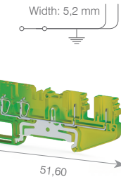
CTP 2.5CT
