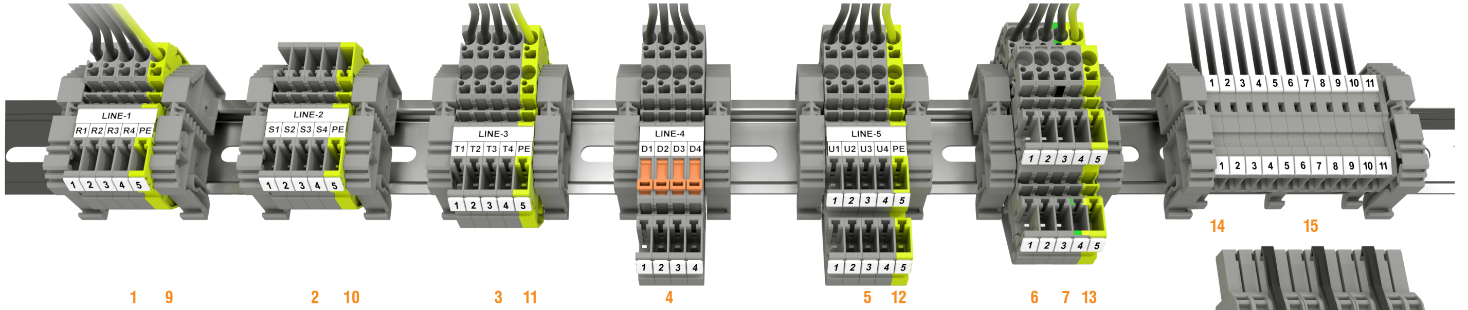
CTP 2.5ET
