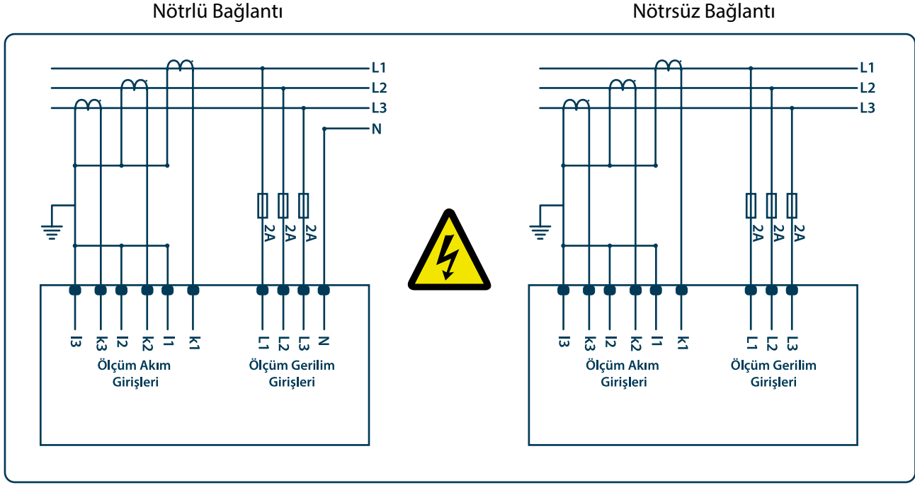
Şekil 2-1 Bağlantı Şemaları
