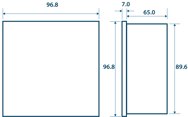
Şekil 2-3 KLEA 220P Boyutlar
